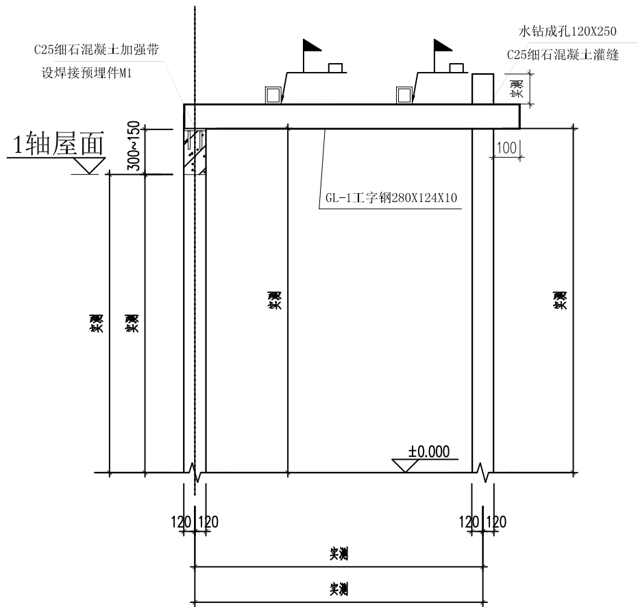
GL-1(GL-2)详图
